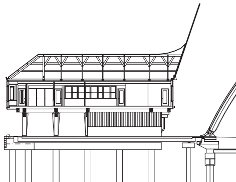
doorsnede
