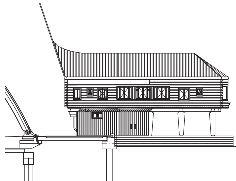
oostgevel
