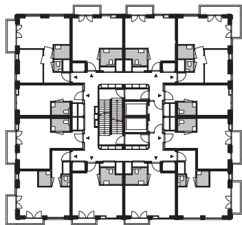
dertiende verdieping
